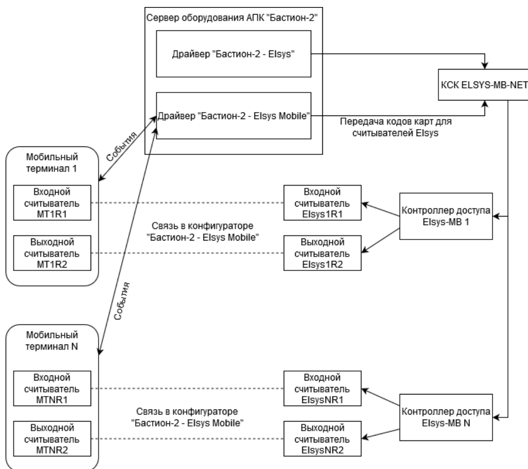
Рис. 2. Использование мобильного устройства в качестве считывателя карт доступа
